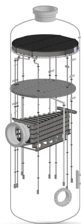
TYPE MV-V
